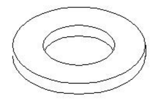
(D)*8 平垫,金属 Φ6*18*1.2 Flat washer, metal Φ6*18*1.2
