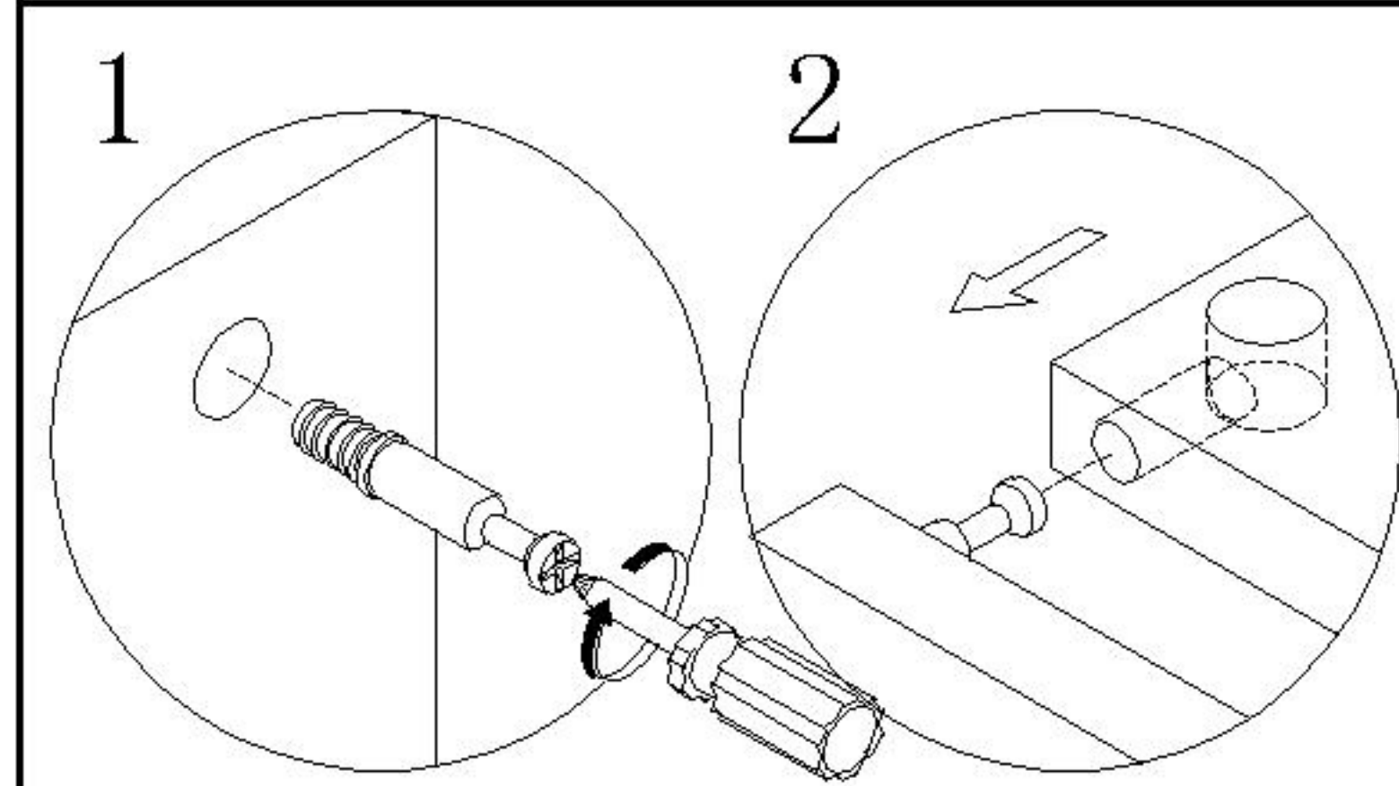
塑料螺母 Plastic Nut
