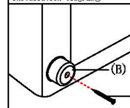
图2: 边脚安装示意图②
